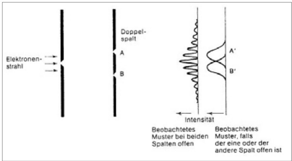
Fig. 3 : Intensitäts-Verteilung von überlagerten Wellen (links) und von Kügelchen (rechts) hinter einem Doppelspalt.
