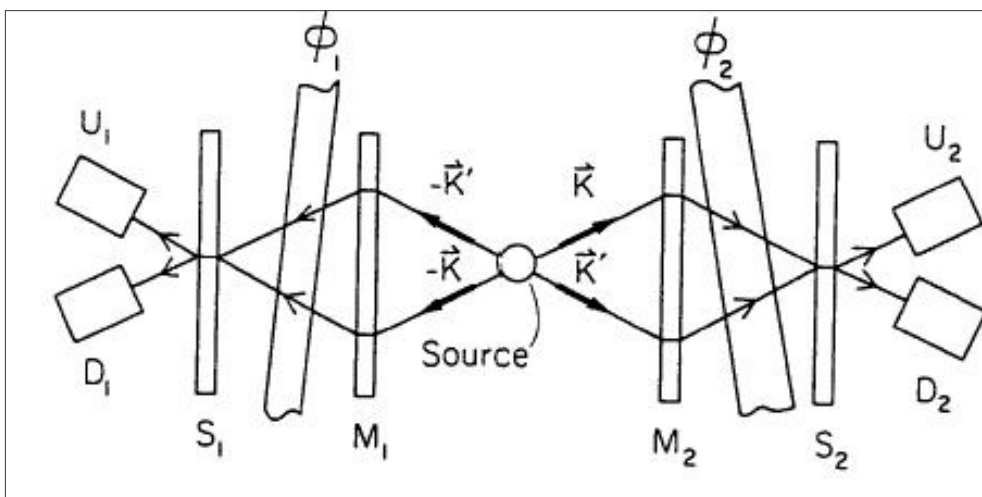
Fig.6: Schema des EPR-Interferometers nach Horne und Zeilinger.
