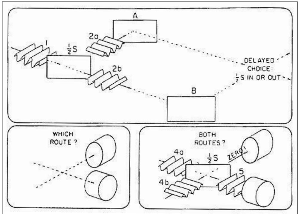
Fig. 4: Schema von Wheeler's „Delayed-Choice Experiment“. (Nach J.A. Wheeler 1988 5 )
